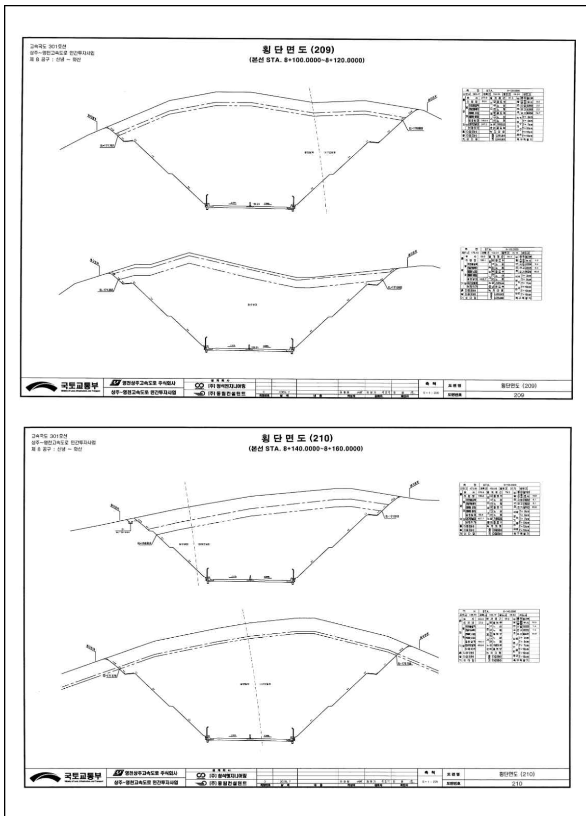
【그림 53.1.5】 표준횡단면도
